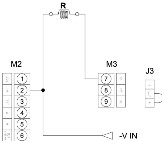
Relè Comune Negativo
