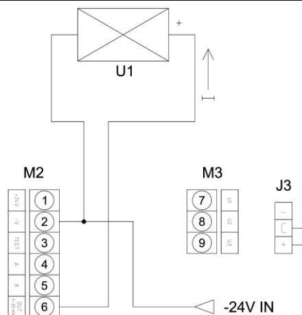
U1 Utilizzatore Ad Esempio PLC
