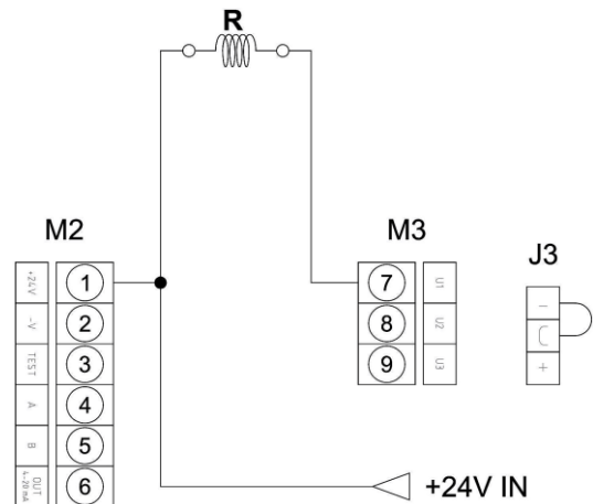
Relè Comune Positivo
