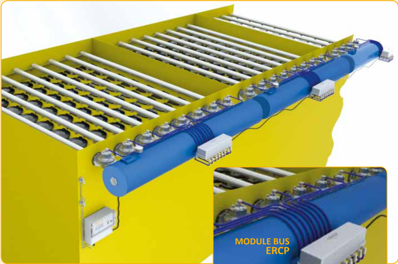
RACCORDEMENT ÉLECTROPNEUMATIQUE DES VALVES
