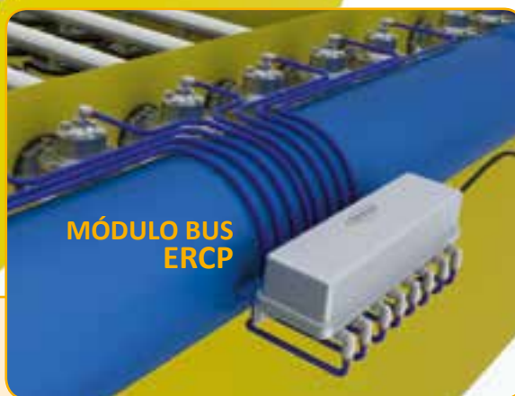
CONEXIÓN ELECTRONEUMÁTICA DE LAS VÁLVULAS
